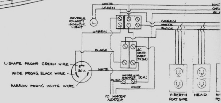
DETAIL A- 110 V WIRING S
